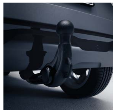
▲ Tažné zařízení Včetně 13pólové elektroinstalace. Pevné, odnímatelné, vyklápěcí.
